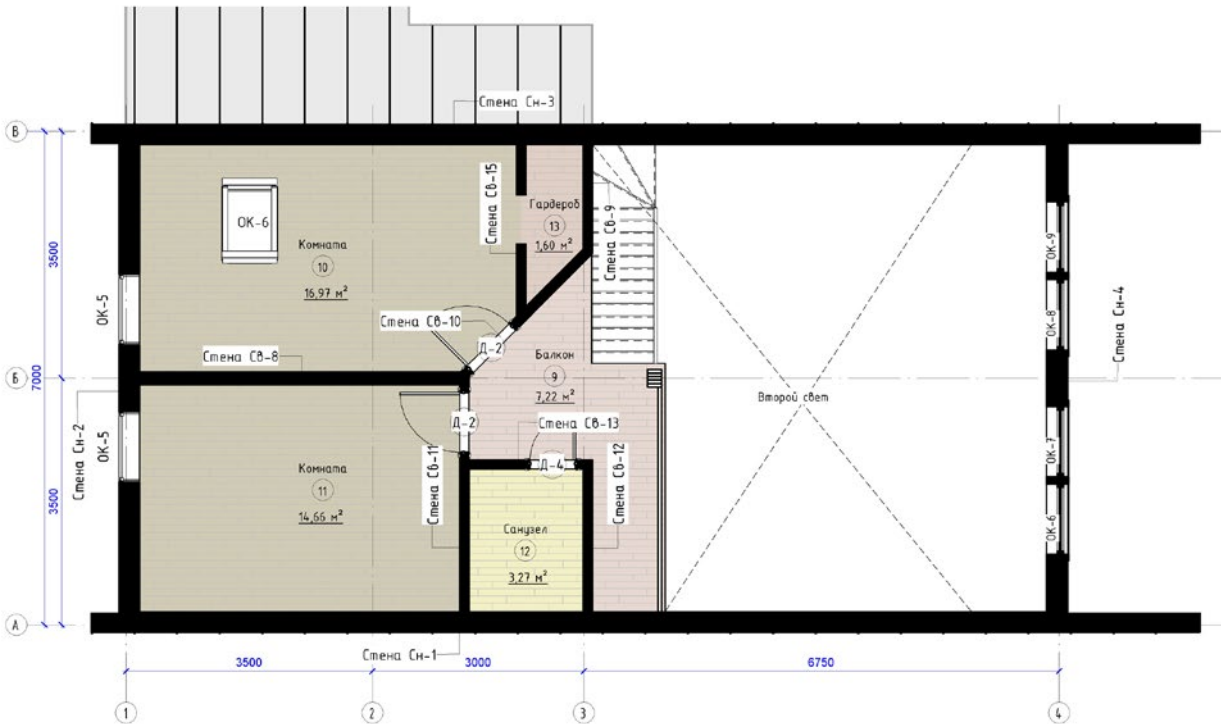
Маркировочный план 2 эт. 1 : 50
